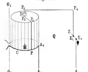
Detail zur Versuchsordnung Einthovens.
